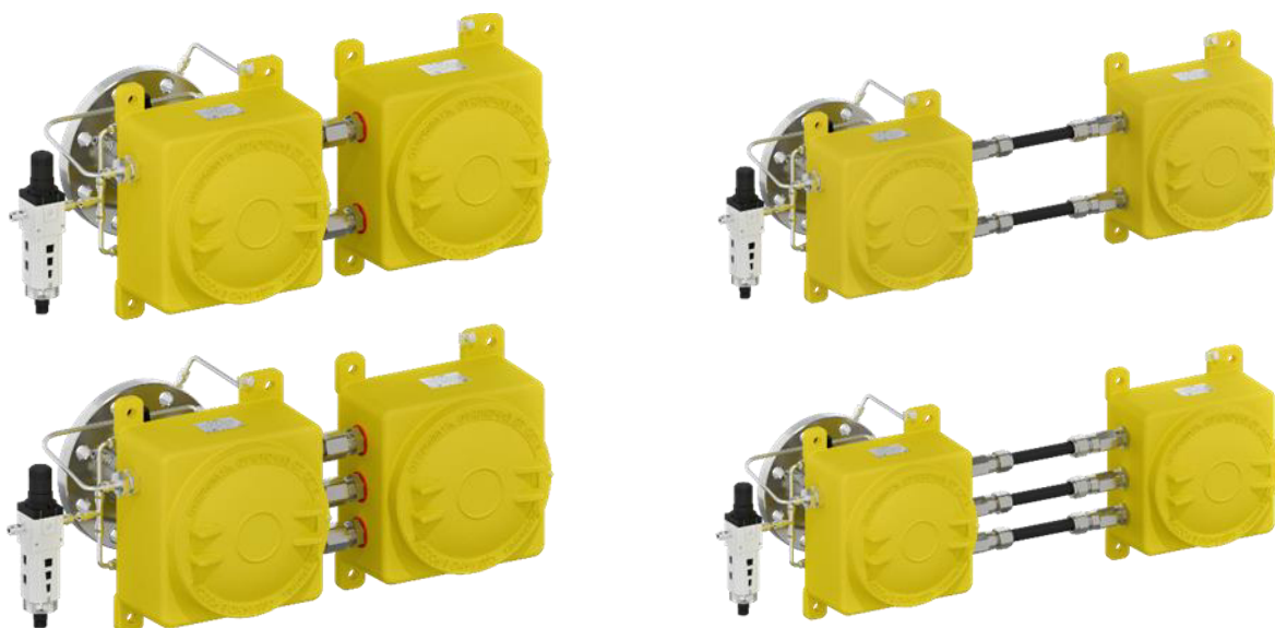
Рисунок 2 – Общий вид измерительного блока газоанализаторов стационарных ЭРИС Оксидиркон 2, ЭРИС Оксидиркон 3, ЭРИС Оксидиркон 4; слева - жесткое соединение сенсорного и электронного блоков, справа - разделенное
