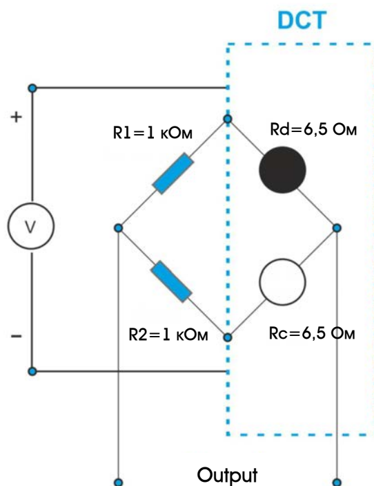
Схема подключения DCT серия 4R
