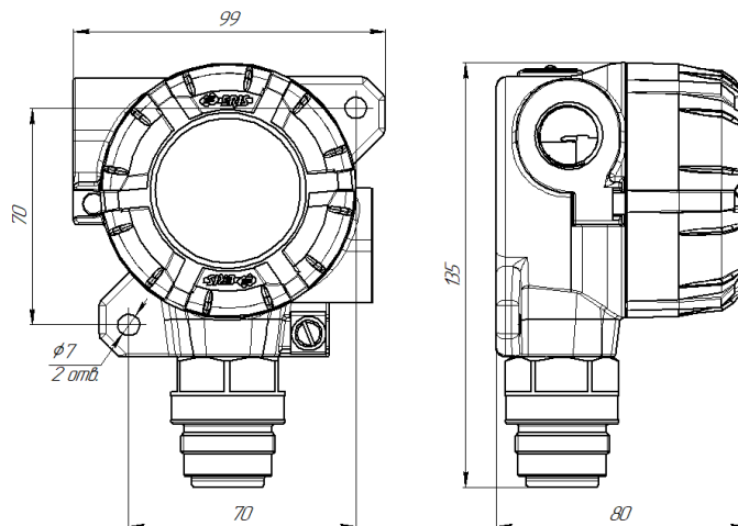
Рисунок 3– Габаритные размеры ERIS XS HT
