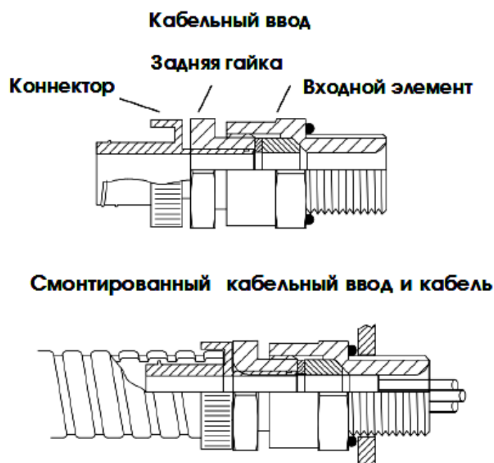
Рисунок 5 – Монтаж кабельного ввода
