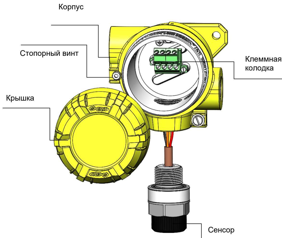
Рисунок 17 – Замена сенсора
