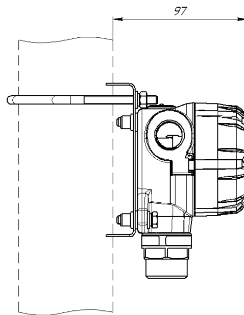
Рисунок 11 – Вид датчика, установленного на трубу
