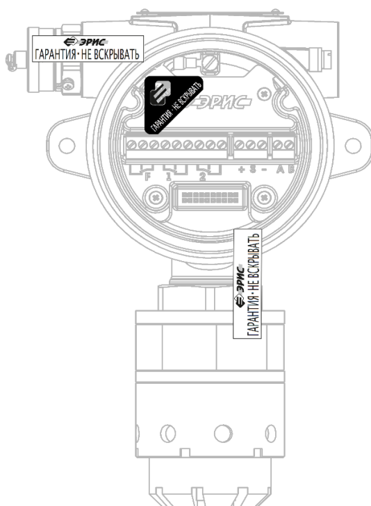
Рисунок 7 - Места нанесения пломб
