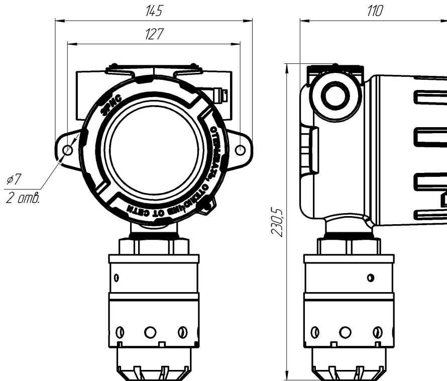
Рисунок 3 – Габаритные размеры ДГС ЭРИС-ФИД в корпусе типа А
