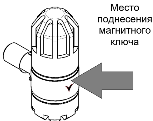
Рисунок 31 – Место поднесения магнита к CZO
