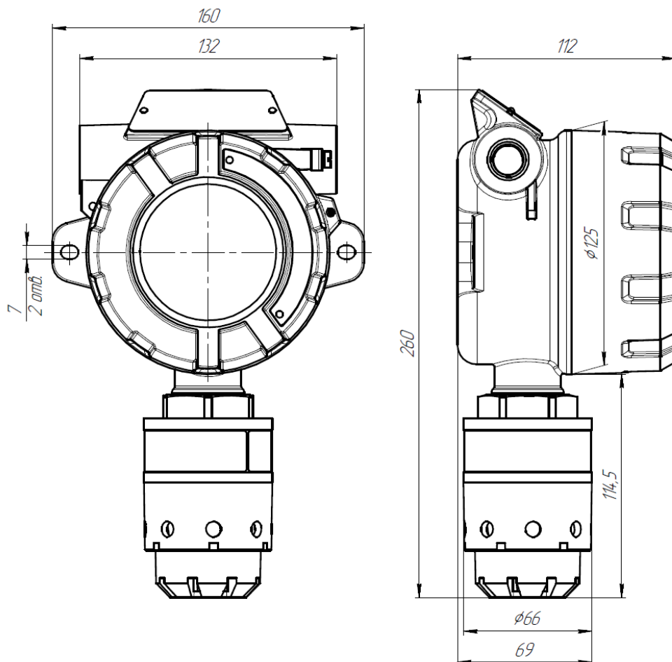
Рисунок 4 – Габаритные размеры ДГС ЭРИС-ФИД в корпусе типа Б
