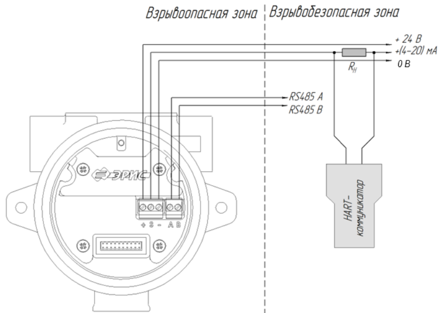
Рисунок 17 – 3-проводная схема подключения газоанализатора ДГС ЭРИС-ФИД без реле с подключением HART по токовой петле ( R_n = 250 \text{ Ом} )
