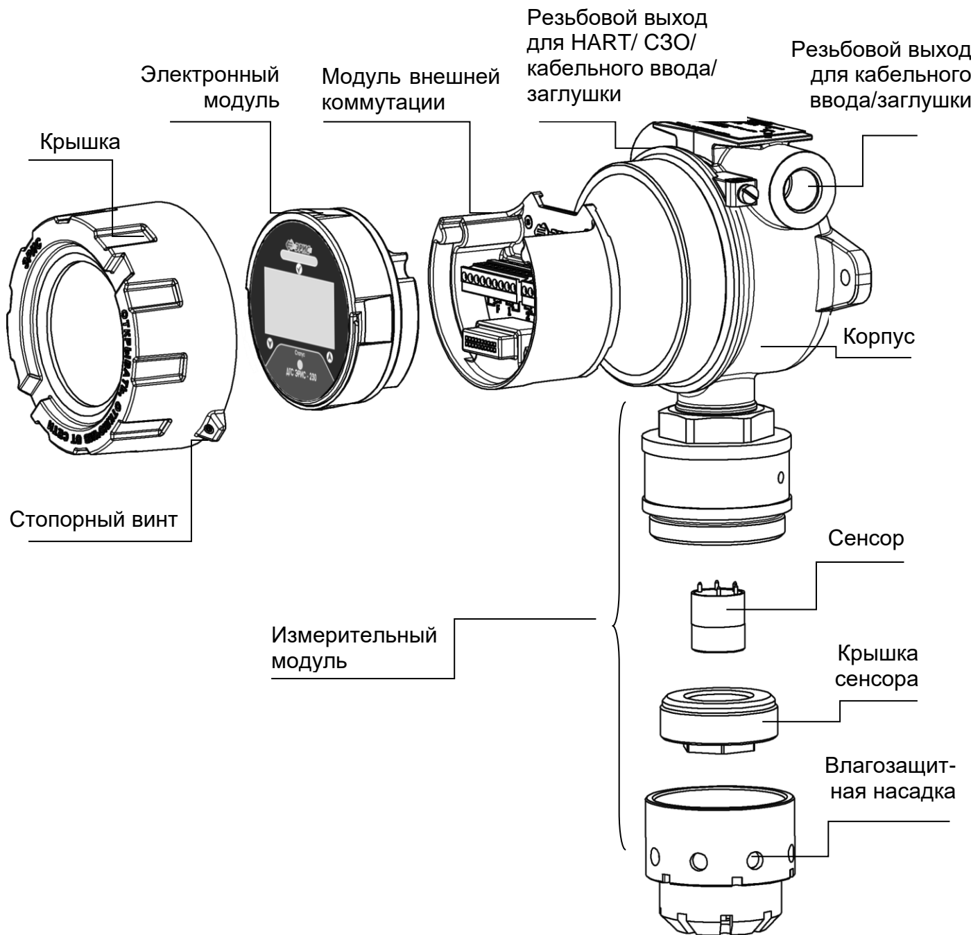
Рисунок 5 – Функциональный состав ДГС ЭРИС-ФИД
