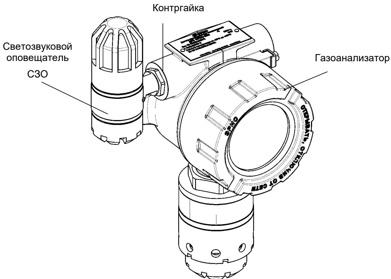
Рисунок 30 – Внешний вид газоанализатора со светозвуковым оповещателем CZO
