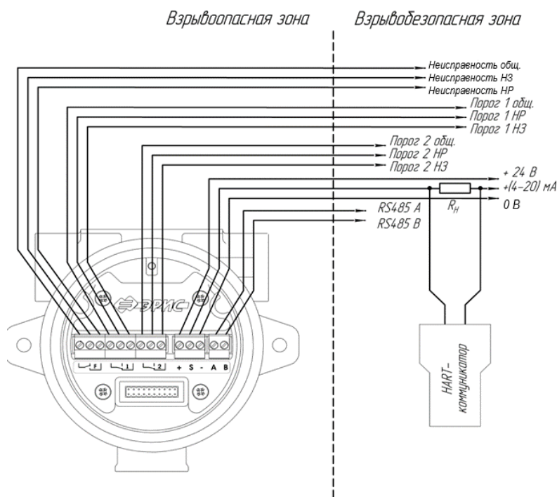
Рисунок 18 – 3-проводная схема подключения газоанализатора ДГС ЭРИС-ФИД с реле с подключением HART по токовой петле. НР - нормально разомкнутый контакт; НЗ - нормально замкнутый контакт. ( R_n = 250 \text{ Ом} )
