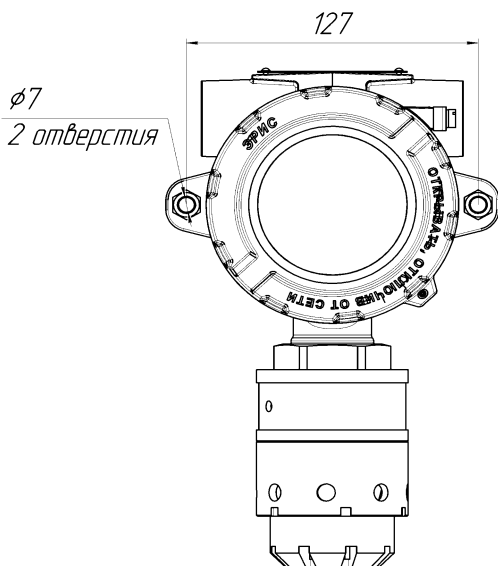
Рисунок 8 – Монтажные размеры
