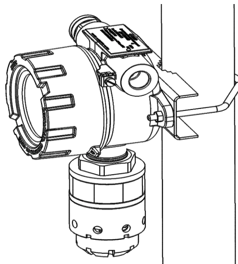
Рисунок 11 – Вид газоанализатора, установленного на трубу
