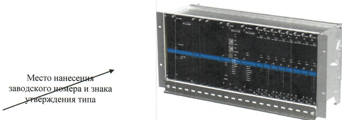
Рисунок 6 – Общий вид контроллеров модели ЭРИС-2100
