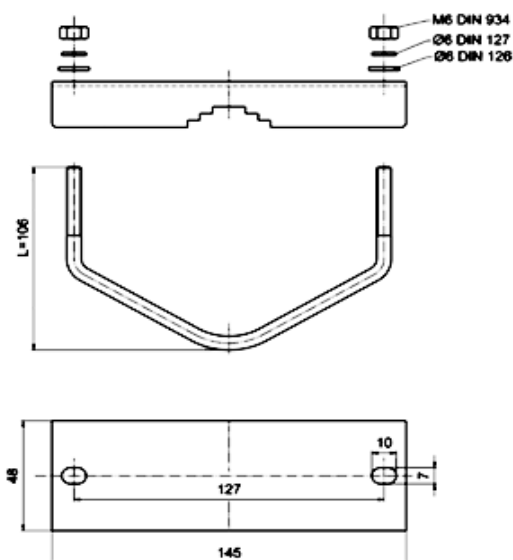
Рисунок 10 – Вид крепления для установки на трубу
