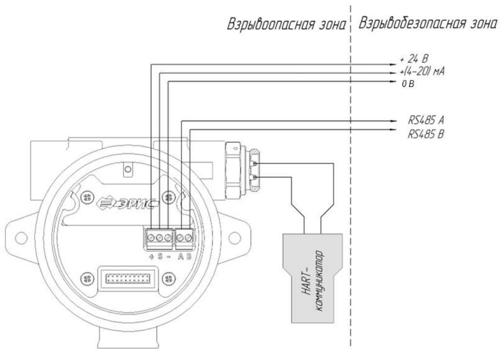
Рисунок 19 – 3-проводная схема подключения газоанализатора ДГС ЭРИС-230 без реле и с подключением локального HART
