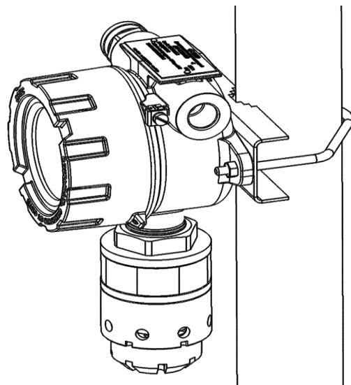
Рисунок 11 – Вид газоанализатора, установленного на трубу
