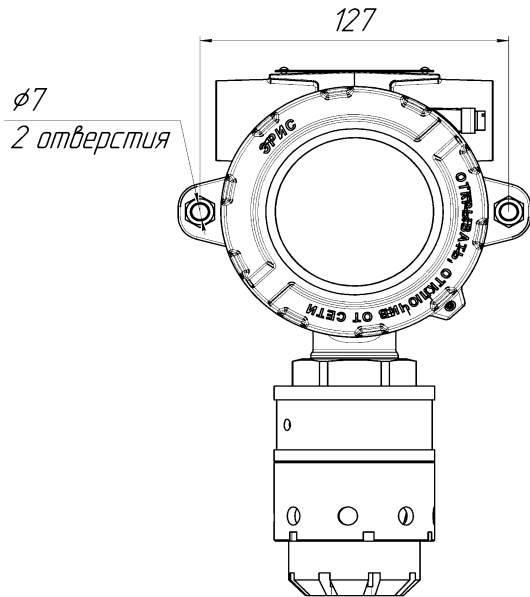
Рисунок 8 – Монтажные размеры
