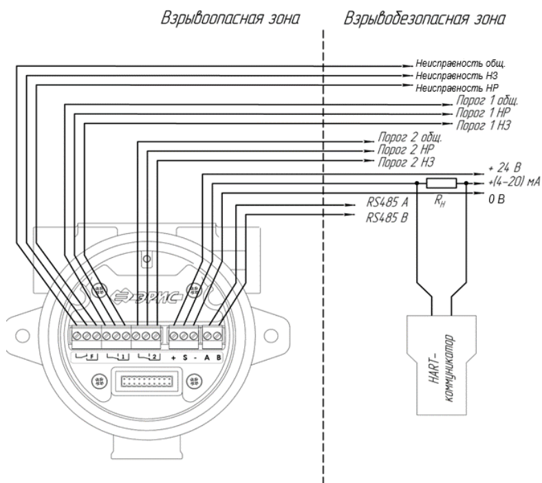
Рисунок 18 – 3-проводная схема подключения газоанализатора ДГС ЭРИС-230 с реле с подключением HART по токовой петле. НР - нормально разомкнутый контакт; НЗ - нормально замкнутый контакт.
