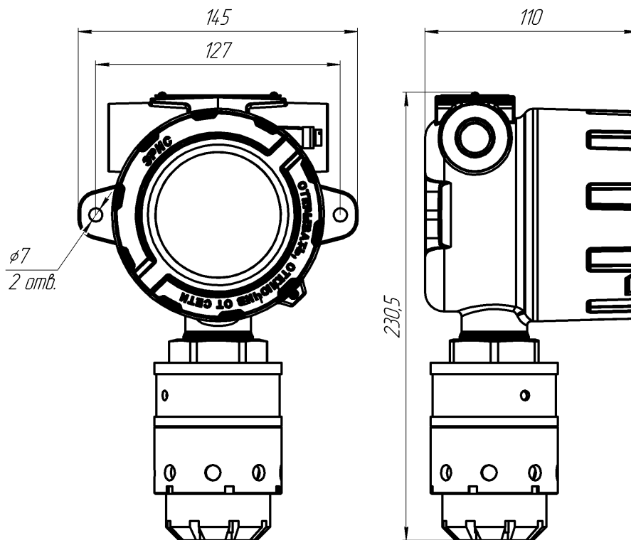
Рисунок 3 – Габаритные размеры ДГС ЭРИС-230 в корпусе типа А
