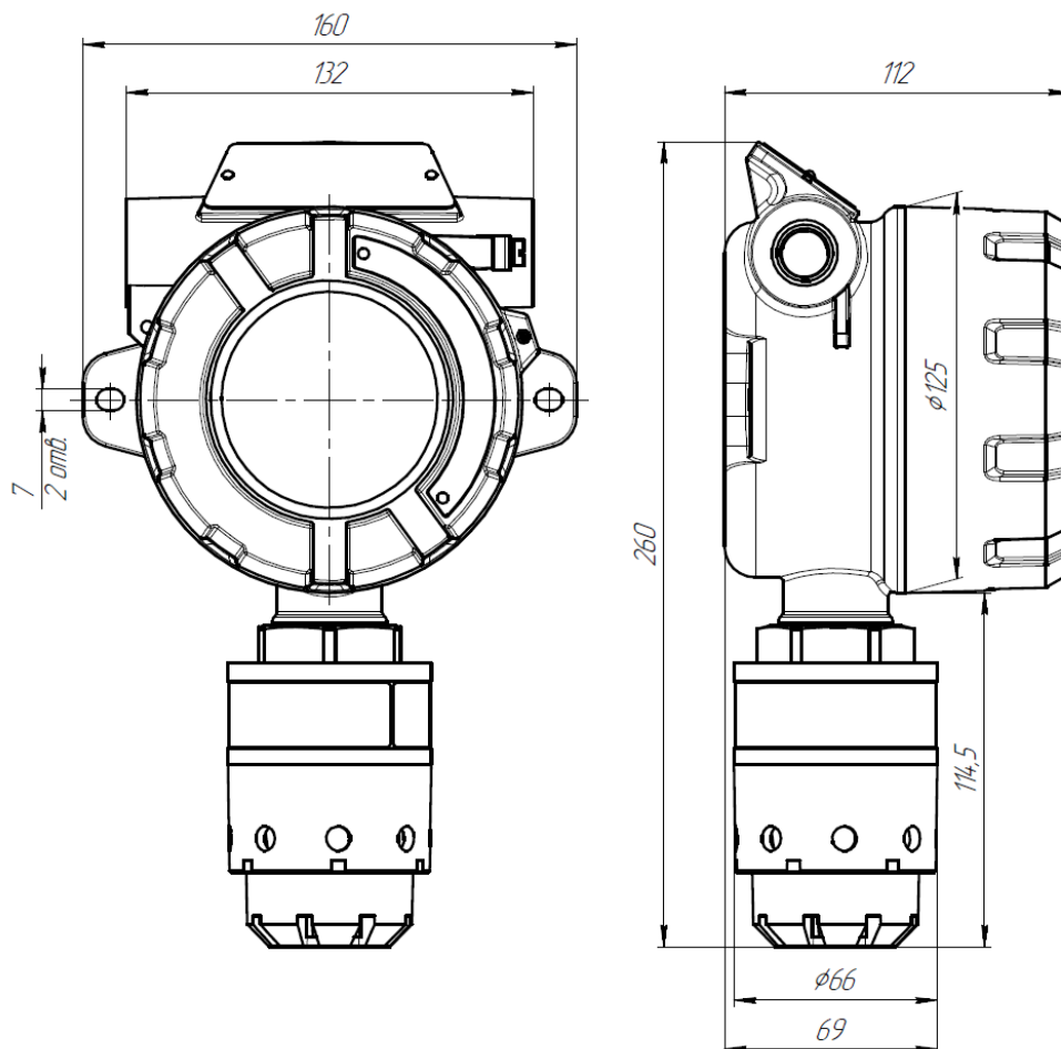
Рисунок 4 – Габаритные размеры ДГС ЭРИС-230 в корпусе типа Б
