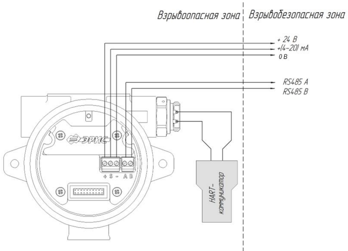
Рисунок 19 – 3-проводная схема подключения газоанализатора ДГС ЭРИС-ФИД без реле и с подключением локального HART
