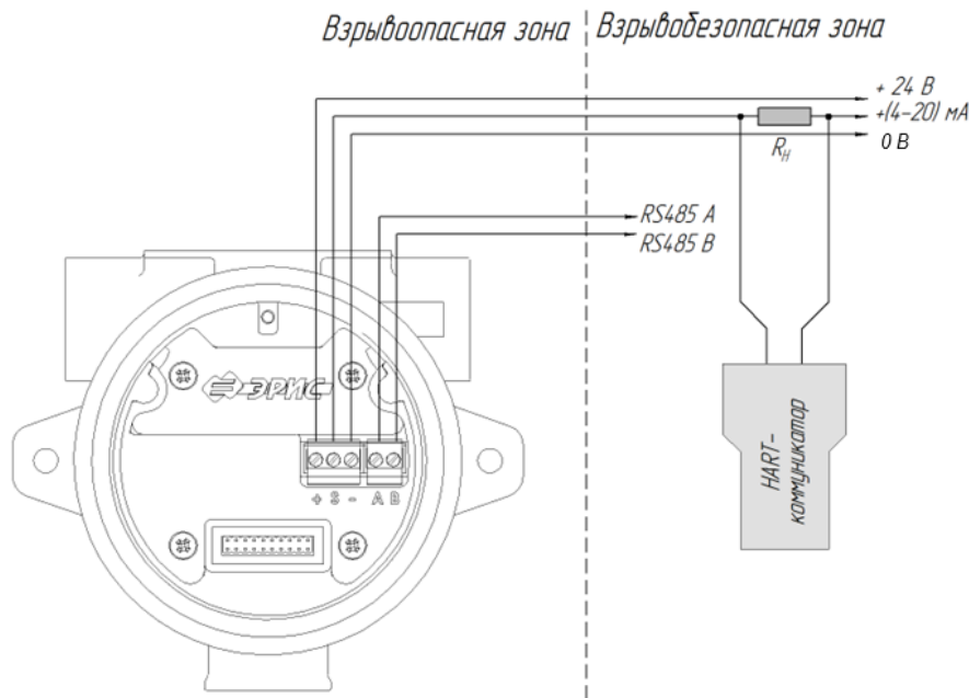
Рисунок 17 – 3-проводная схема подключения газоанализатора ДГС ЭРИС-ФИД без реле с подключением HART по токовой петле
