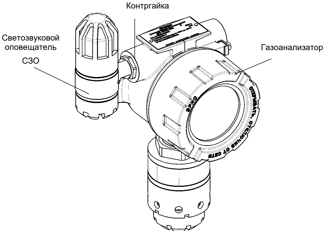
Рисунок 26 – Внешний вид газоанализатора со светозвуковым оповещателем C30
