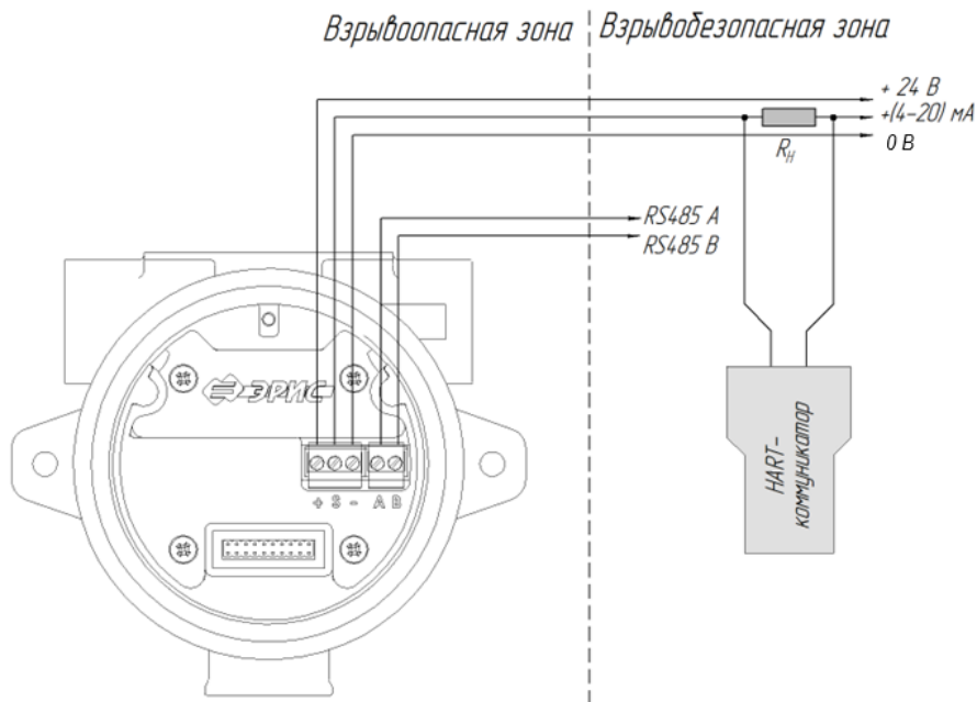
Рисунок 17 – 3-проводная схема подключения газоанализатора ДГС ЭРИС-ФИД М без реле с подключением HART по токовой петле
