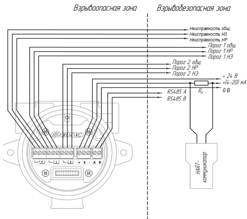
Рисунок 18 – 3-проводная схема подключения газоанализатора ДГС ЭРИС-ФИД М с реле с подключением HART по токовой петле. НР - нормально разомкнутый контакт; НЗ - нормально замкнутый контакт.
