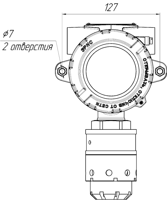
Рисунок 8 – Монтажные размеры
