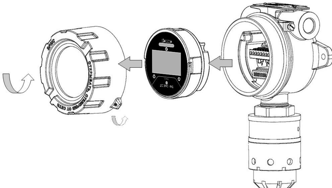
Рисунок 16 – Схема разбора ДГС ЭРИС-ФИД М
