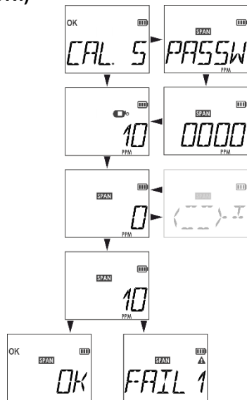
Рисунок 5 – Калибровка диапазона
