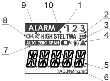
Рисунок 2 – ЖК-дисплей газоанализатора
