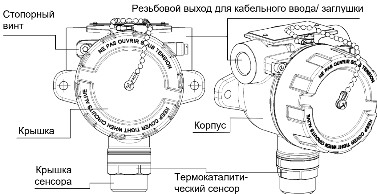
Рисунок 3 – Функциональный состав ERIS XS
