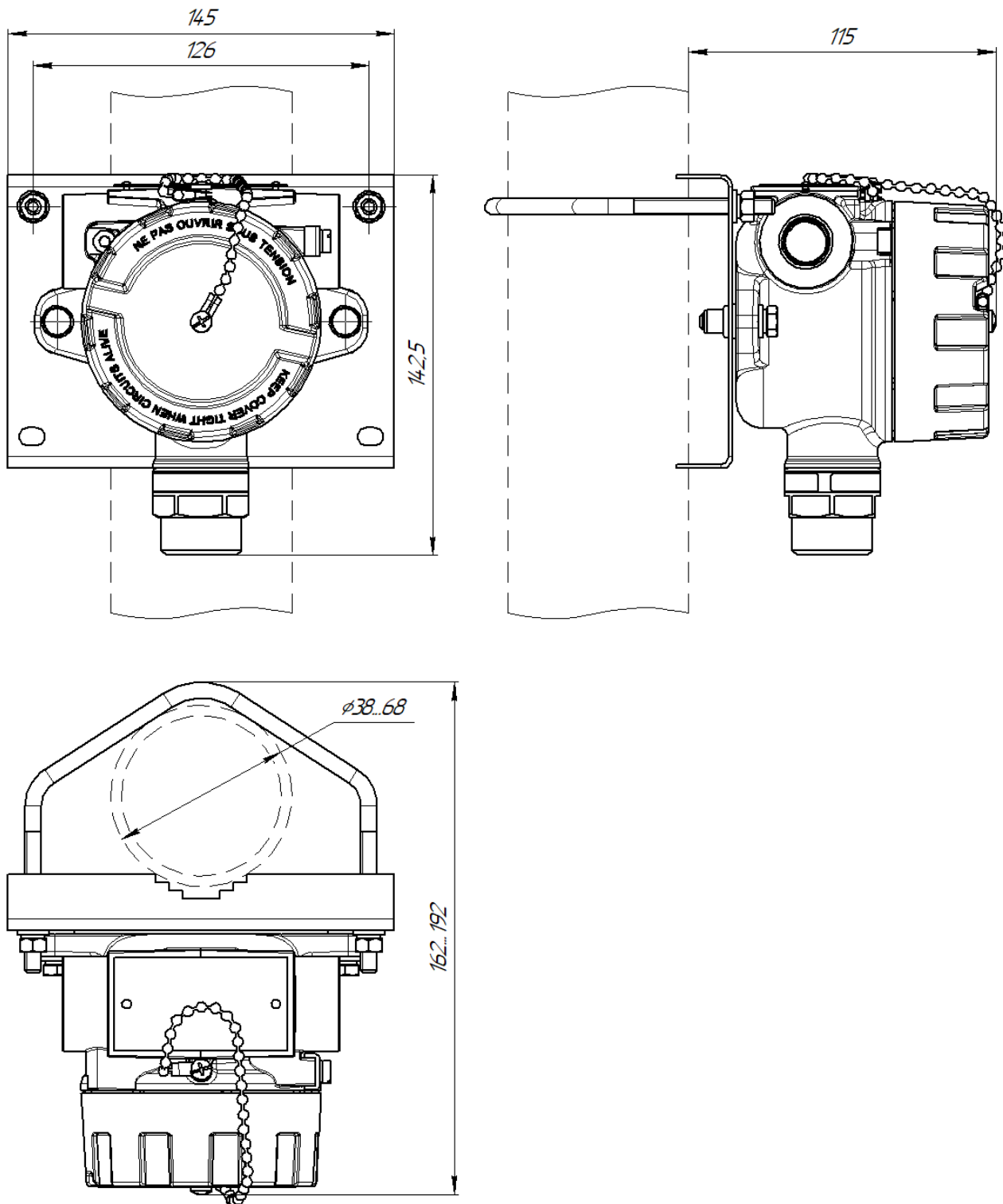
Рисунок 6 – Вид датчика, установленного на трубу
