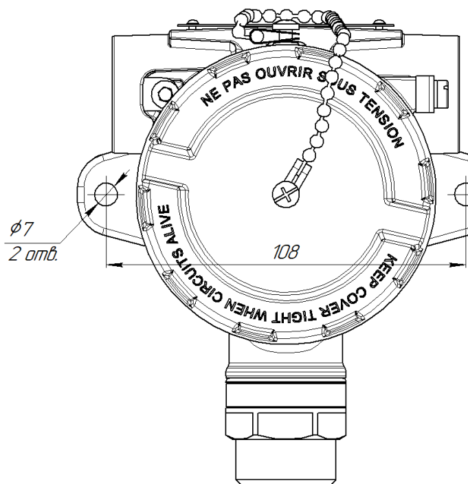
Рисунок 4— Монтажные размеры
