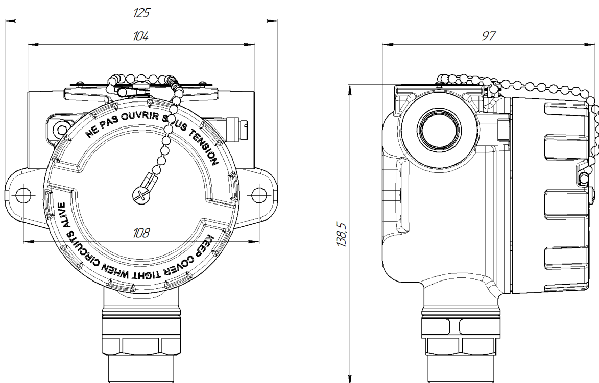
Рисунок 2 – Габаритные размеры ERIS XS
