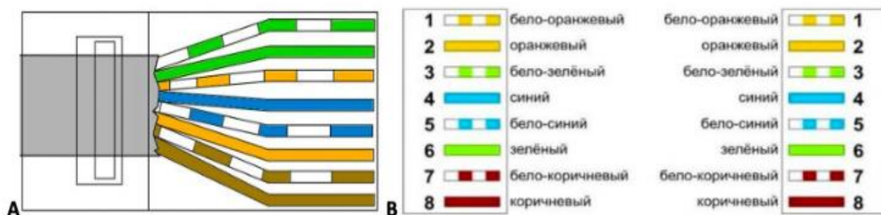
Рисунок В.1 – Разводка сетевого кабеля
