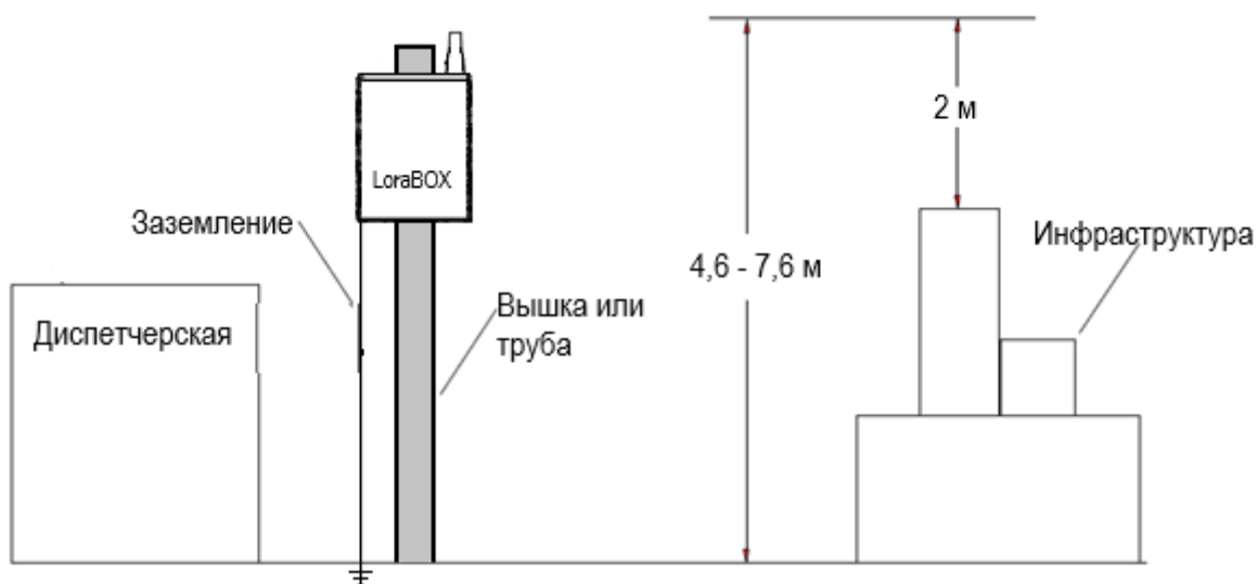
Рисунок 7 – Пример установки LoraBOX
