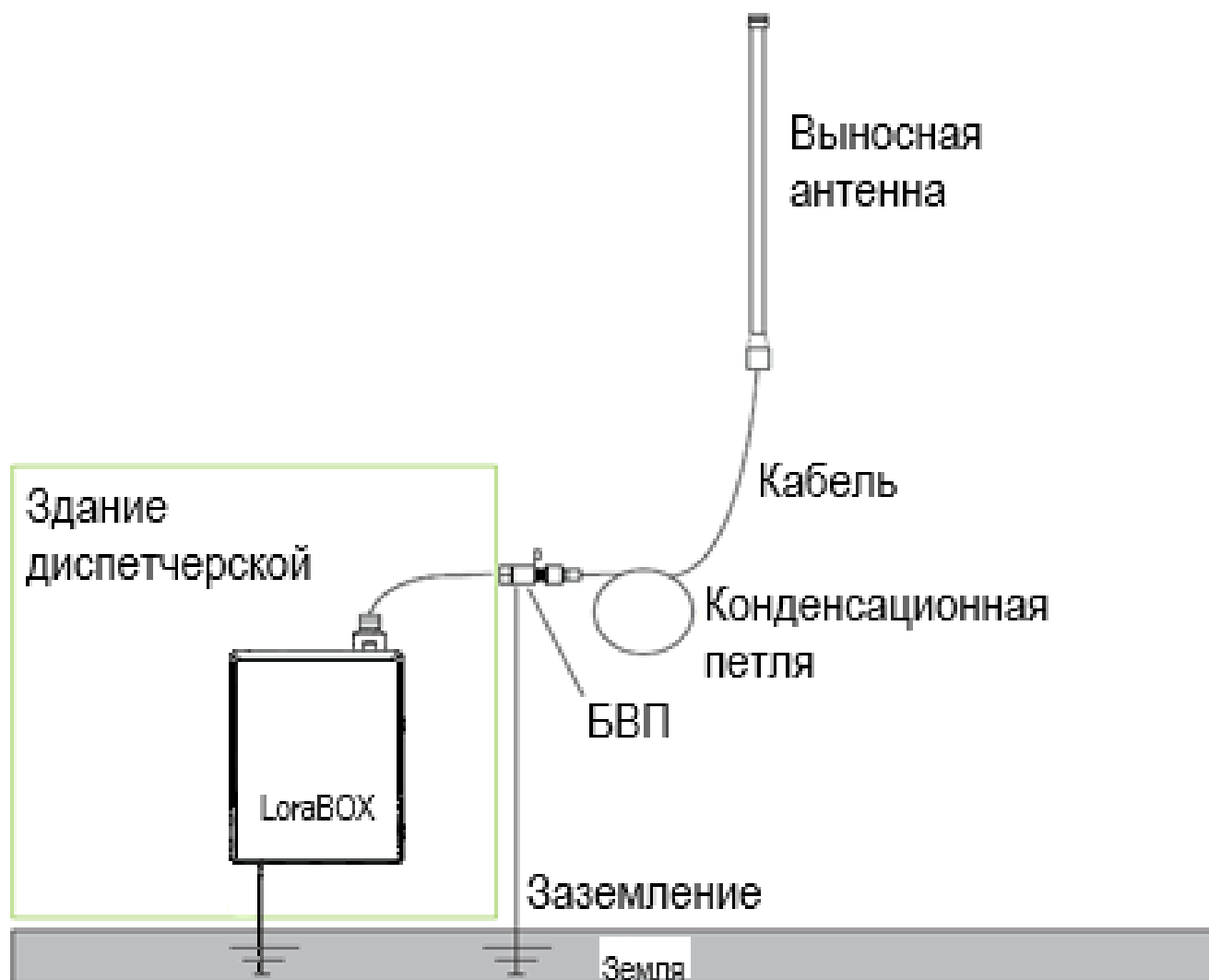
Рисунок А.2 – Схема подключение LoraBOX в помещении
