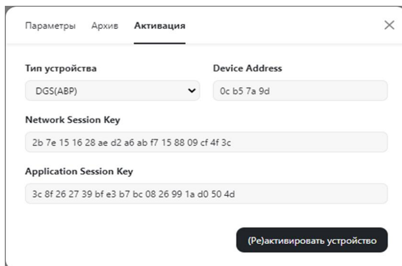
Рисунок 14 – Вкладка Активация
