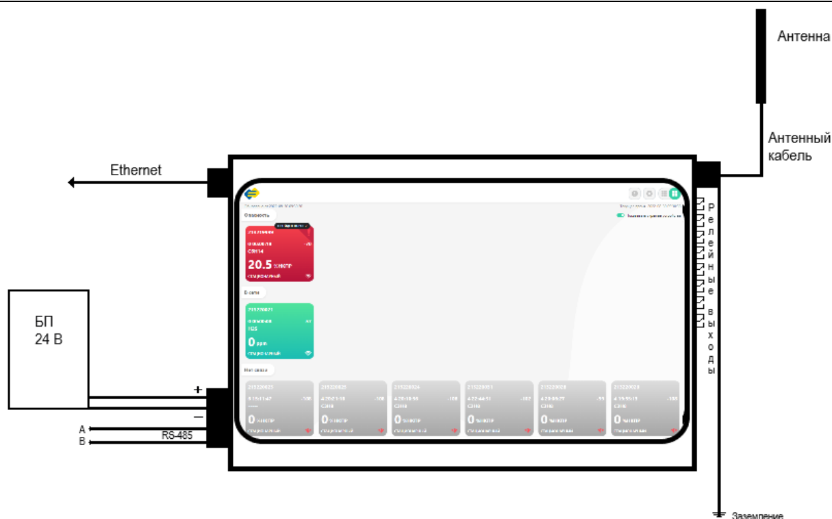
Рисунок 6 – Подключения LoraBOX для проверки работоспособности
